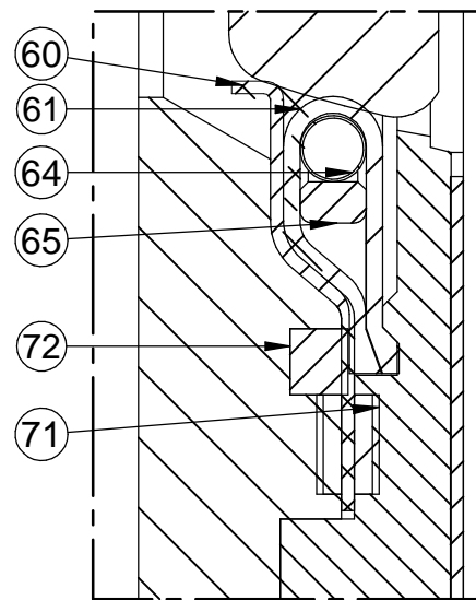
DETALLE - DETAIL B 2:1
