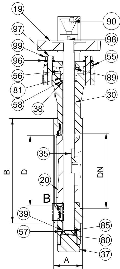
SECCION - SECTION A-A
